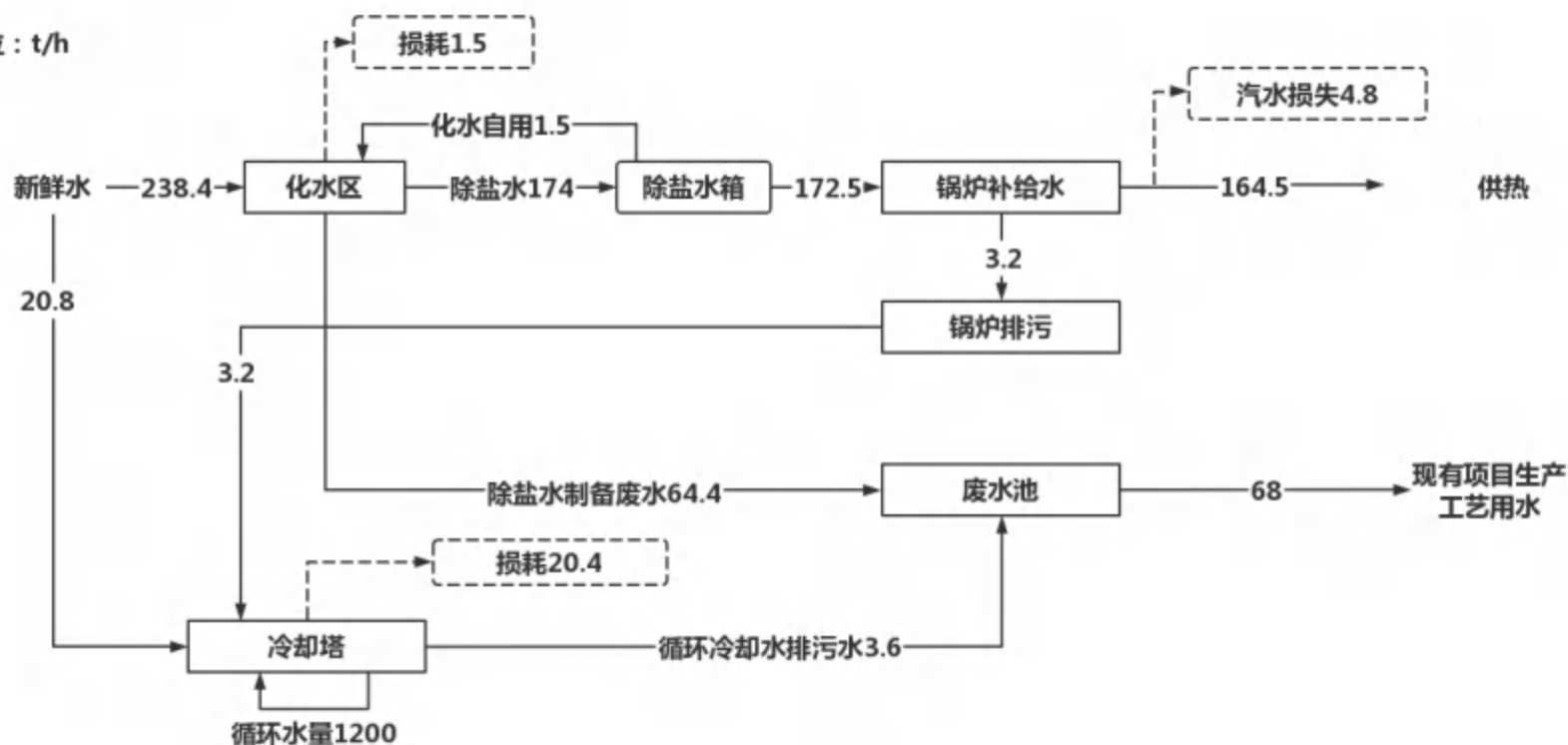
图 2-3 项目水平衡示意图
