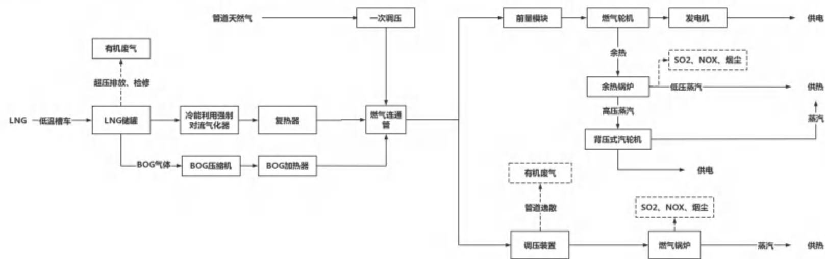
图 2-4 主要工艺流程图
