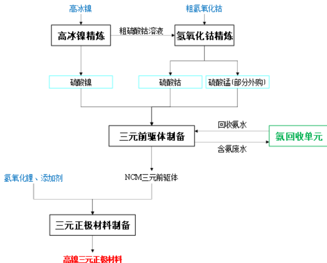
图 2-6 现有项目总体工艺路线示意图
